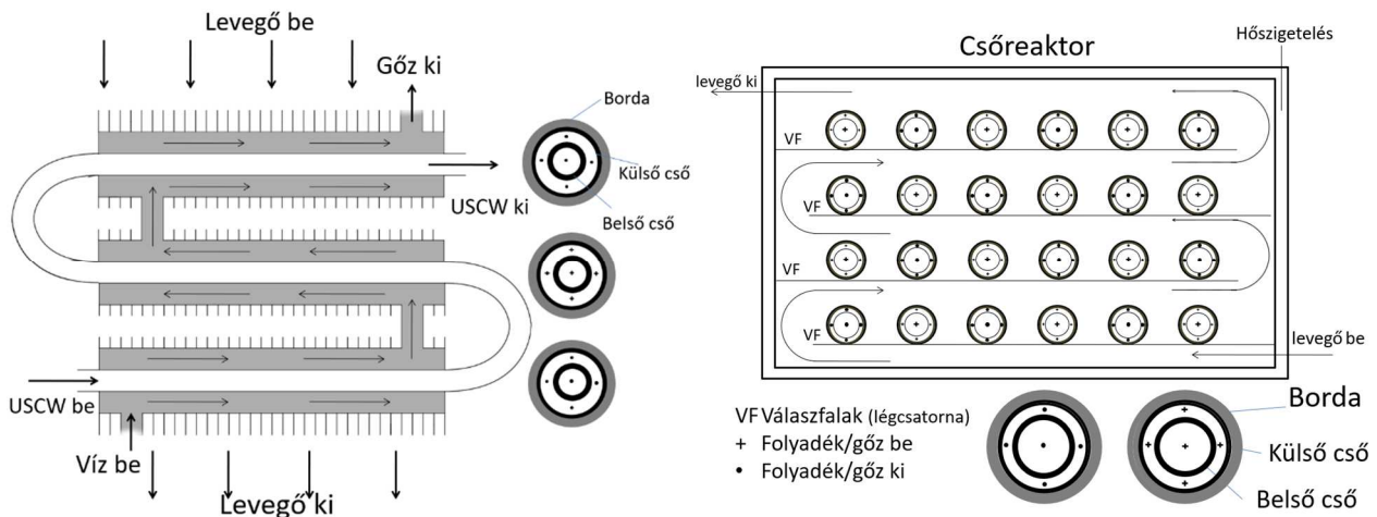
2. ábra. A szuperkritikus üzemű csőreaktor felépítése (bal: főnézetben, jobb: keresztmetszetben)
